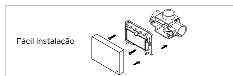
Ilustração de instalação com Mini Neu 2
