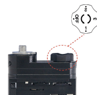
PRO00009 - Plug Altrac PRO com seletor para 3 circuitos
